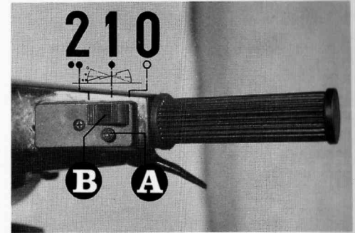
Fig. 19 Conmutador de luces
