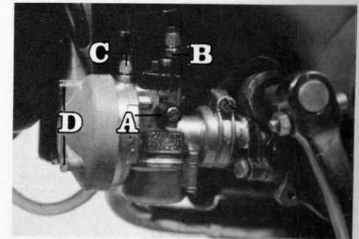
Fig. 26 Ajuste carburación
