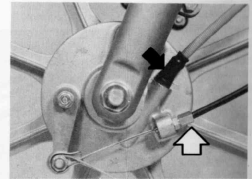
Fig. 29 Regulación de frenos
